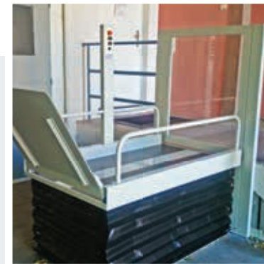
Optionnel: Rampe d'accès prolongée avec portillon supérieur et pilier de contrôle
